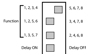
Funkce 5 ON Delay
