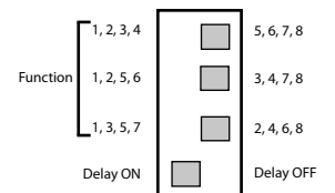
Funkce 8 ON Delay
