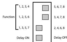
Funkce 7 ON Delay
